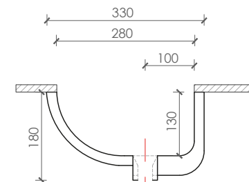
Alzado Lateral
